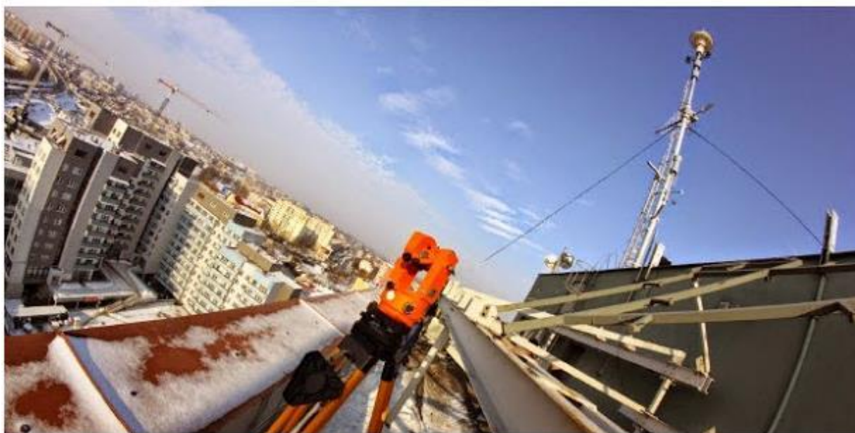
Pomiar pionowości masztu antenowego.
